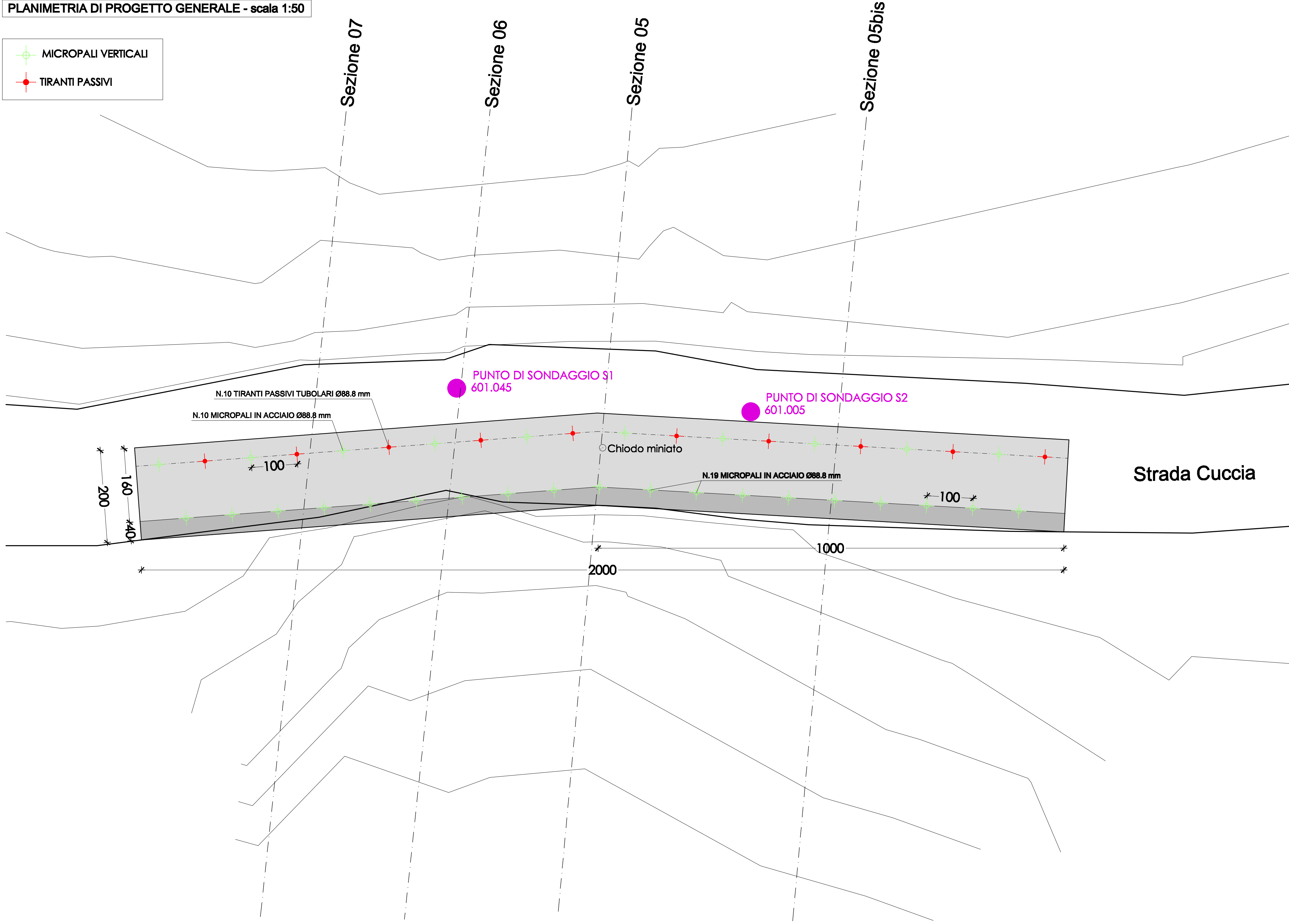
PLANIMETRIA DI PROGETTO GENERALE - scala 1:50
