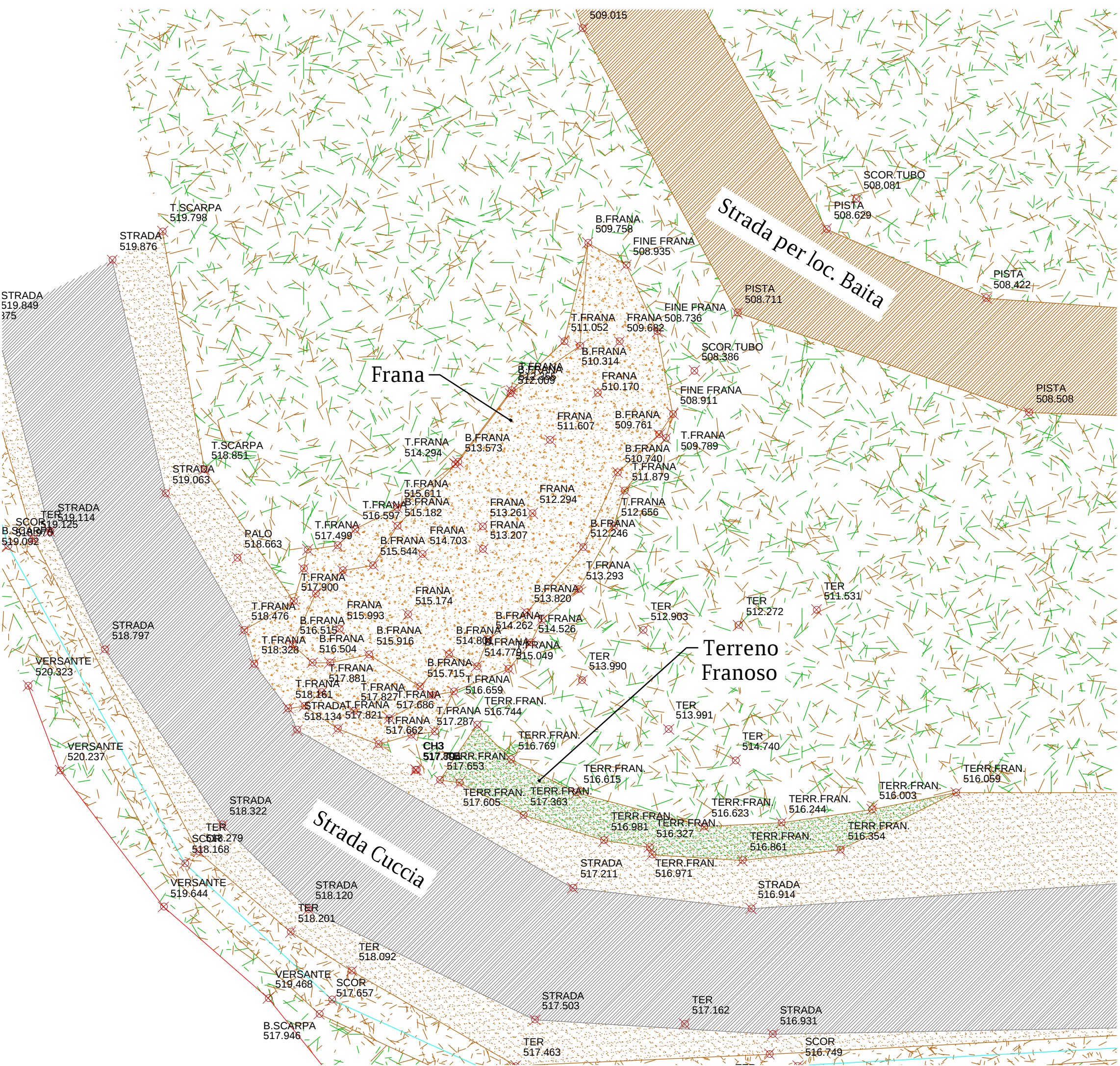
PLANIMETRIA DI RILIEVO INTERVENTO 3 scala 1:100
