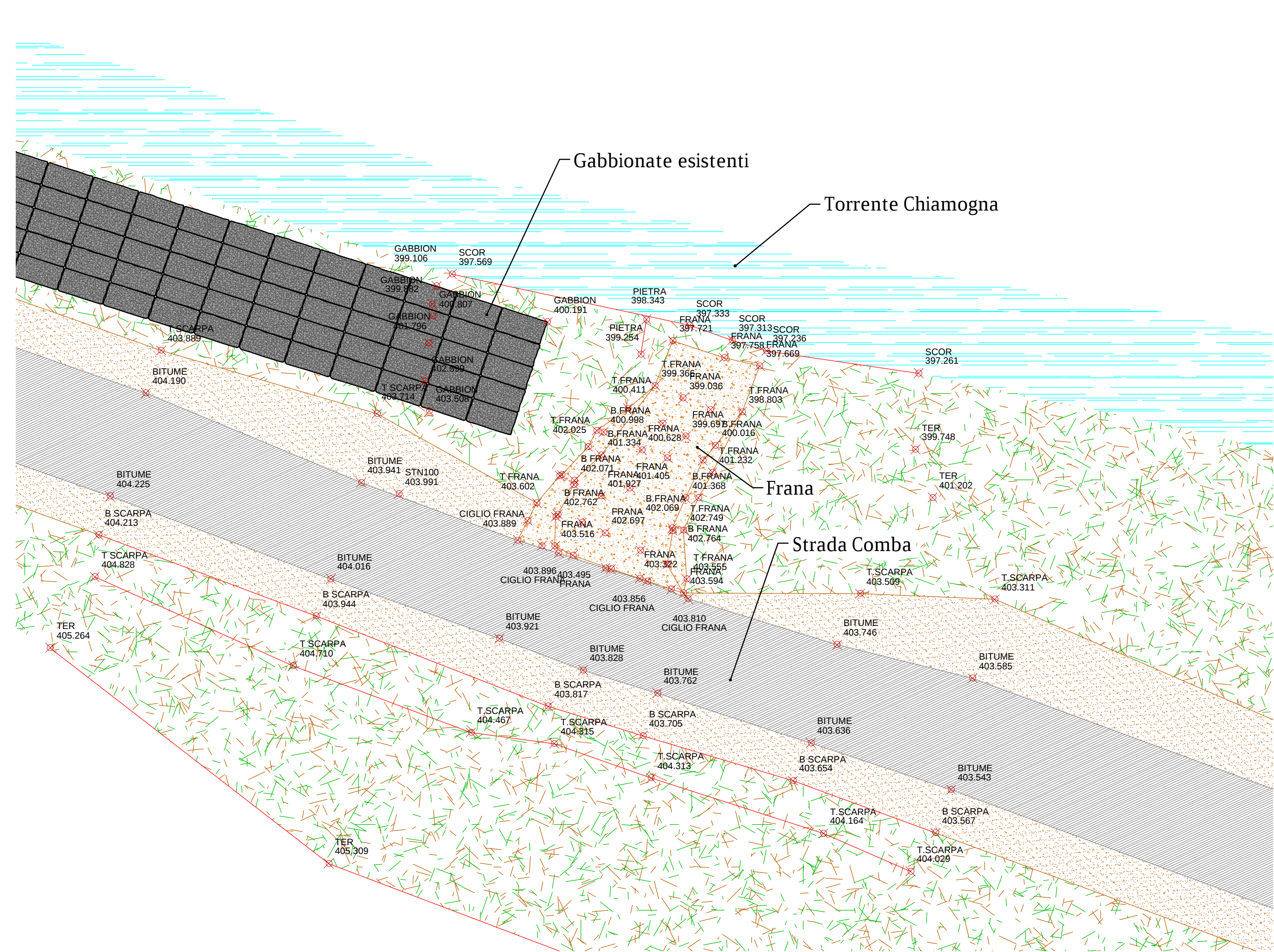
PLANIMETRIA DI RILIEVO INTERVENTO 1 scala 1:100
