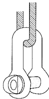
Piegamento della fune su raggio troppo piccolo (in questo caso la portata si riduce a circa il 50%)
