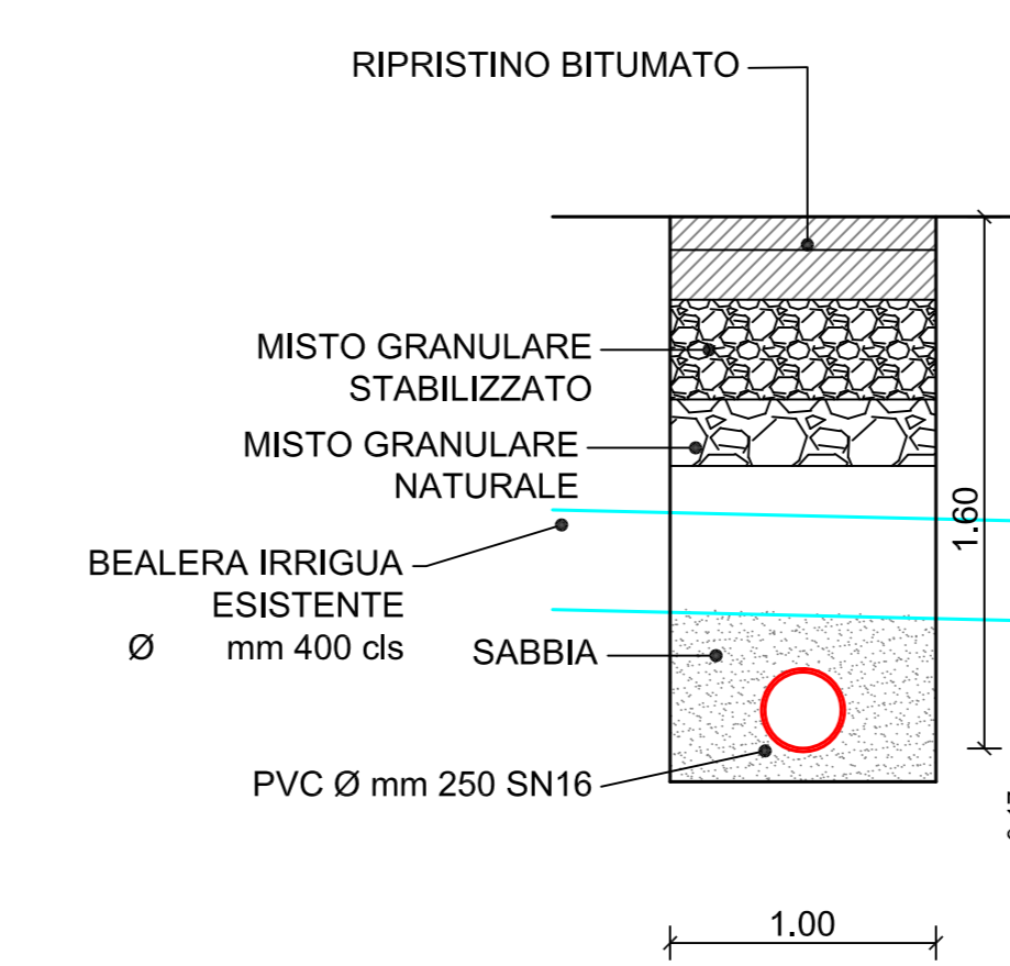
ATTRAVERSAMENTO 4 BEALERA IRRIGUA SCALA 1:25
