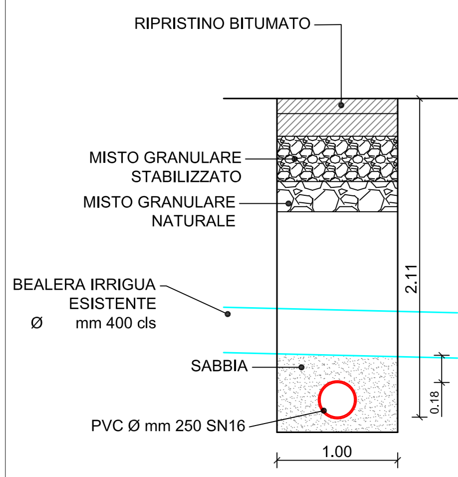
ATTRAVERSAMENTO 1 BEALERA IRRIGUA SCALA 1:25
