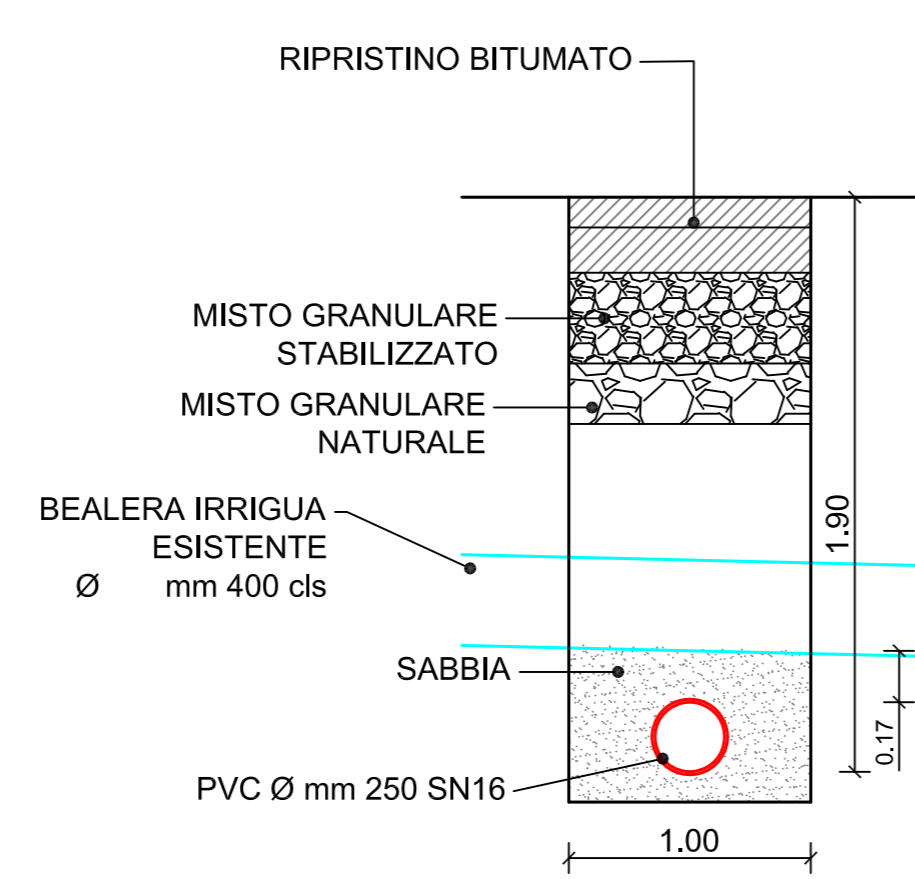
ATTRAVERSAMENTO 2 BEALERA IRRIGUA SCALA 1:25
