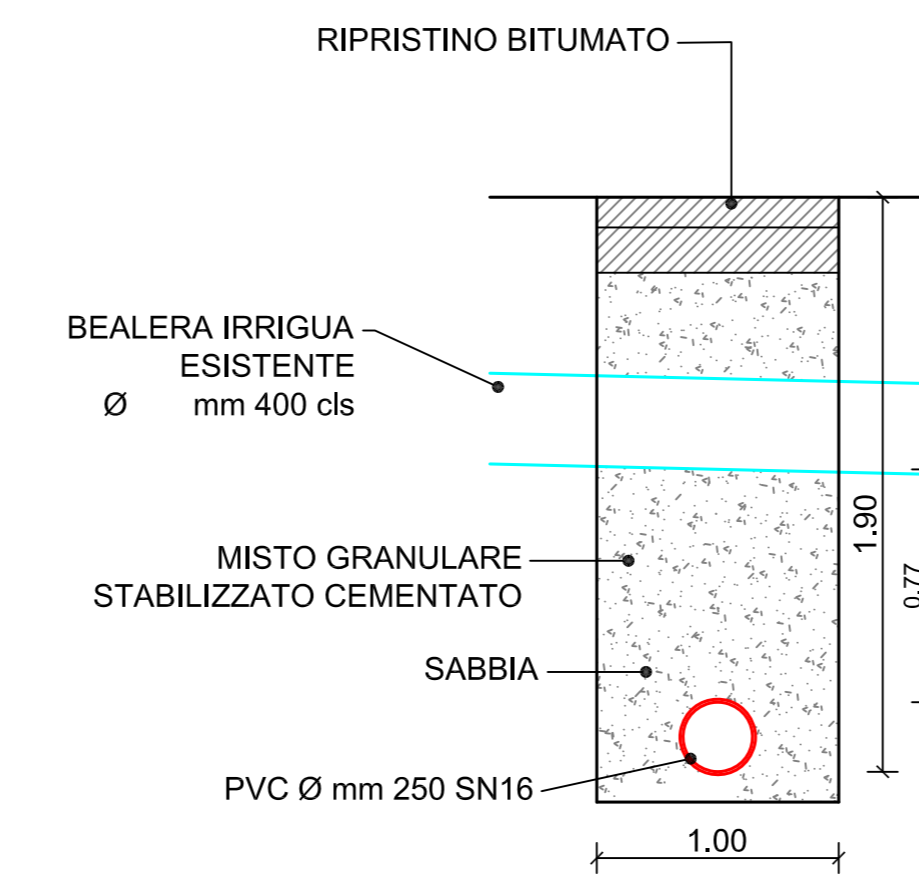
ATTRAVERSAMENTO 3 BEALERA IRRIGUA SCALA 1:25
