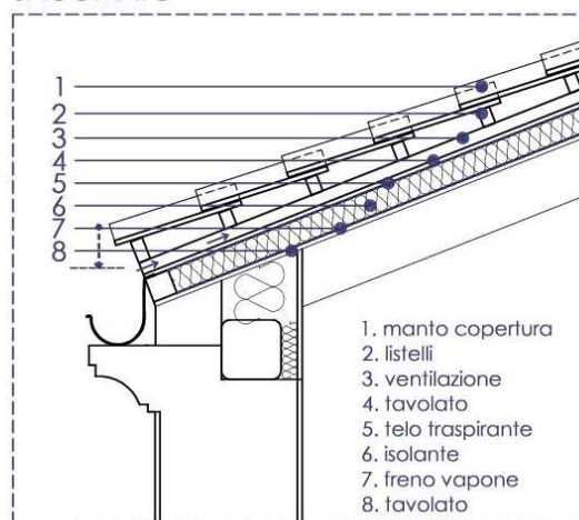
COPERTURA ISOLATA CON CORNICIONE SAGOMATO
