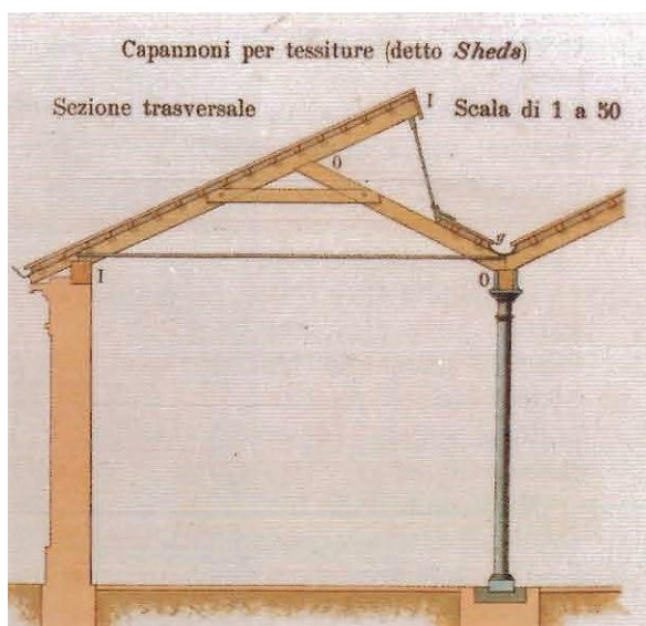
Esempio di copertura in Sheds con struttura lignea e colonne in ghisa
