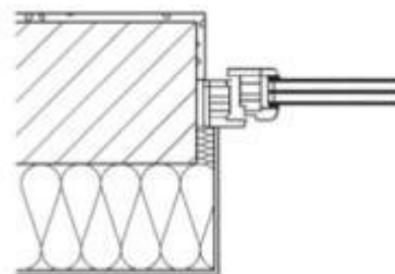
Esempio con risvolto minimo dell'isolante: soluzione da evitare.
