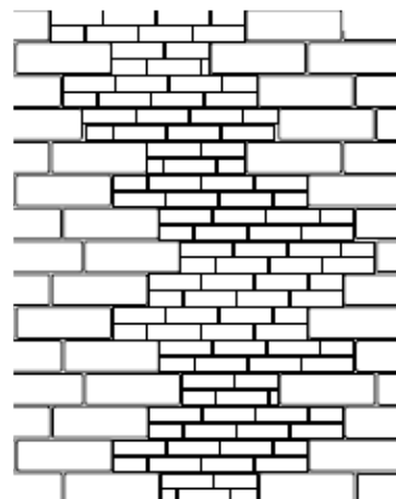
Esempio di paramento murario lesionato. Esempificazione schematica prima e dopo l'intervento
