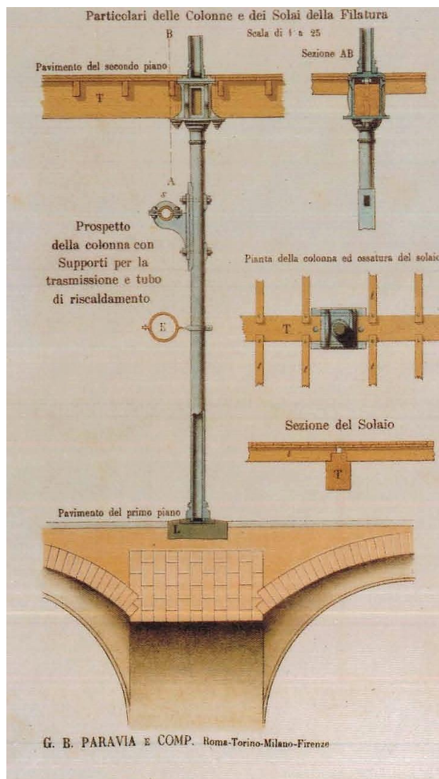
Esempio di colonne in ghisa ed orizzontamenti lignei
