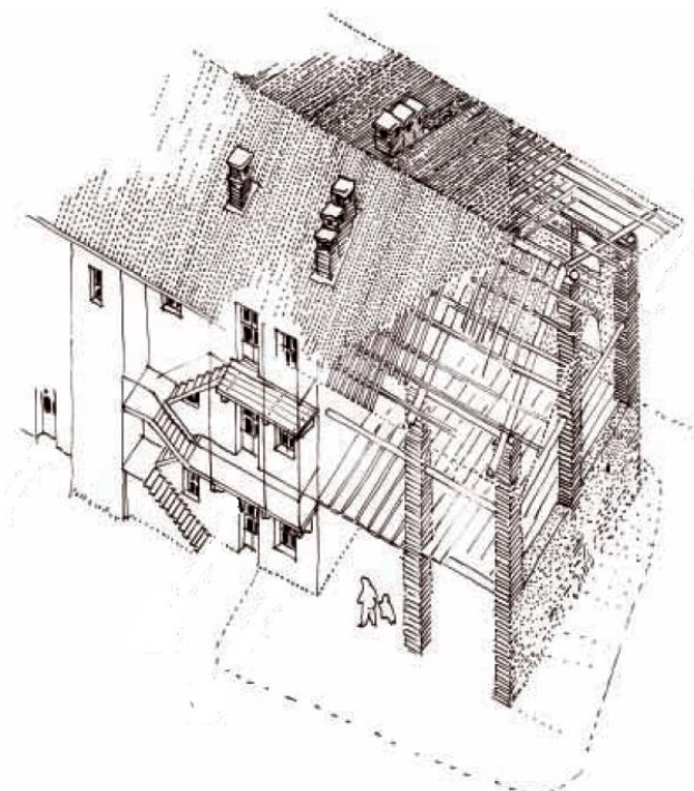
Esempio di cascinale nella sua situazione originale
