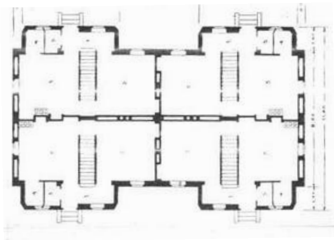
Villaggio "Edoardo Agnelli": Planimetria e immagini odierne della soluzione a quattro alloggi
