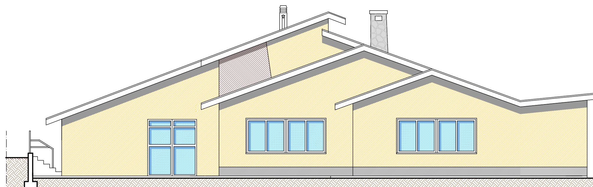
PROSPETTO SUD-OVEST Scala 1:100
